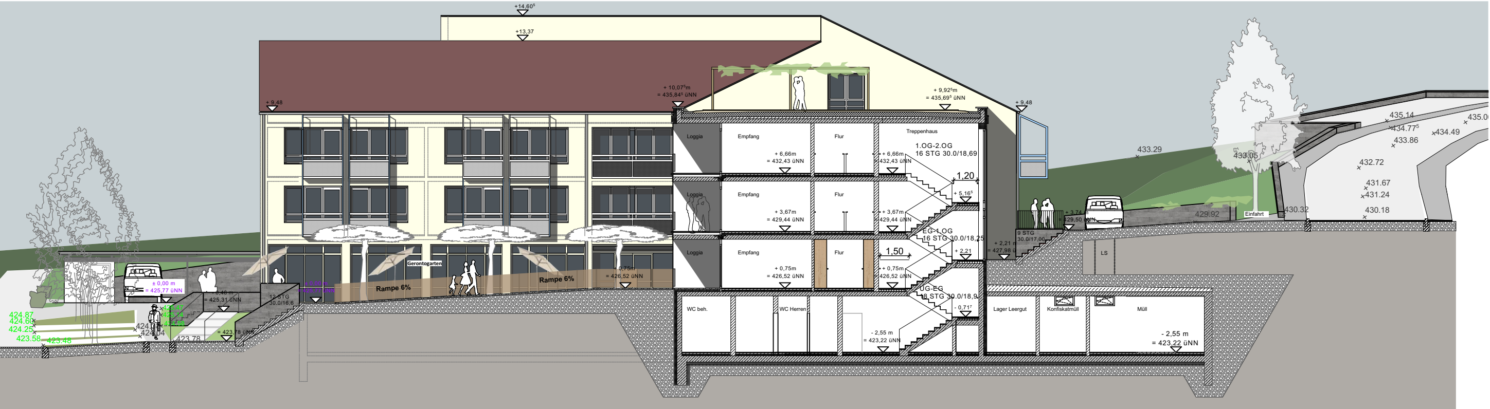
Schnitt E-E
