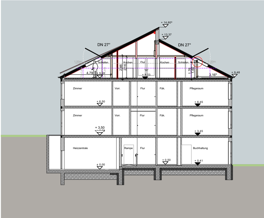
Schnitt D-D
