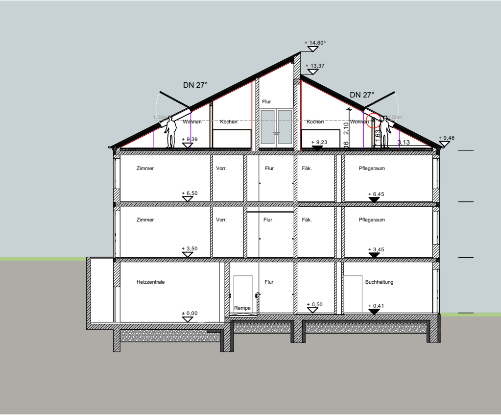
Schnitt B-B
